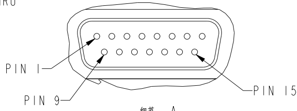
细节 A 比例 1.500
