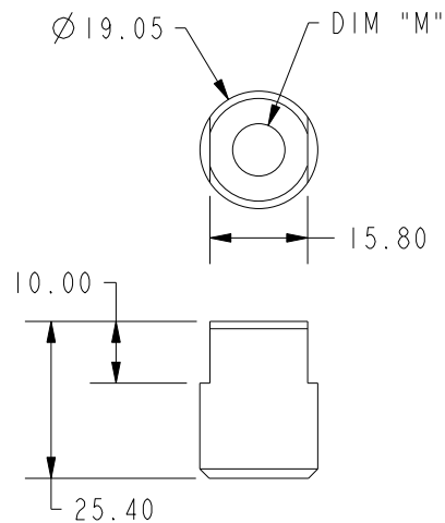
OPTIONAL GEAR SHIFT ADAPTOR 34110-3X
