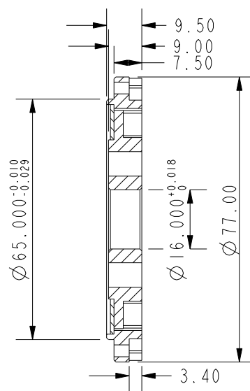
截面 A-A
